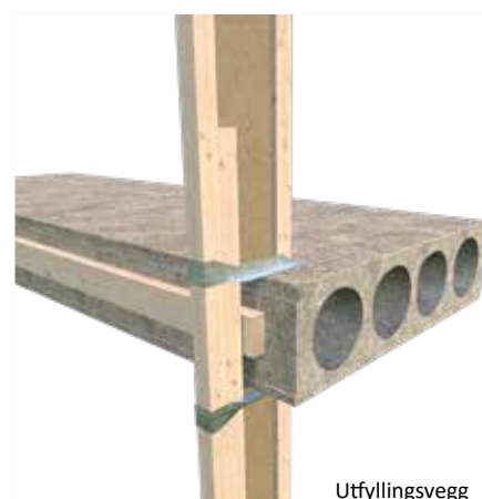
Utfyllingsvegg
