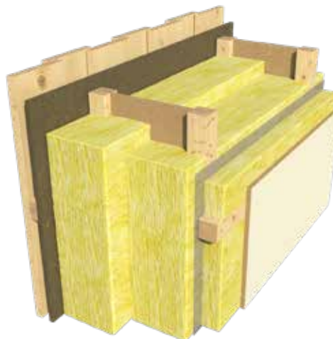
Vegg med 48 mm innføring, med vindspærre av 12 mm trefiberplate.
