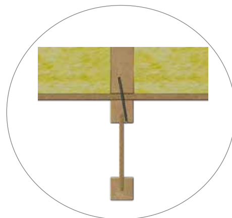
3.3: Innfesting gjennom flens til eksisterende bindingsverk med 5-6 mm treskruer. Benyttes ikke selvborende skruer må flens forbores.
