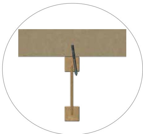
3.1: Innfesting gjennom flens til eksisterende betong og murvegg med betonghylse, ekspansjonsbolt ol. Flens forborres, og det bør ikke benyttes hull diameter større enn 8mm.
