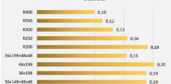
U-verdier i vegg av Masonite- eller heltre stender
